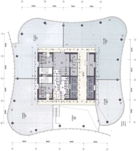
三十七层平面图
